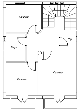
Piano Primo H = 2.80
